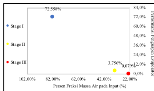
Gambar 3. Grafik Performansi Penguapan
