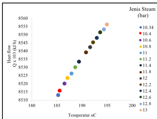
Grafik 4. Perubahan Heat flow yang dihasilkan berbagai jenis steam
