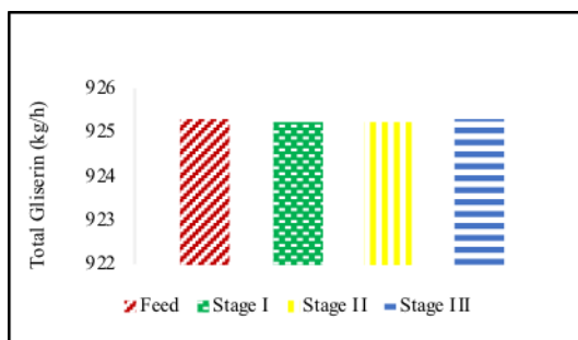
Gambar 1. Grafik Total Gliserin tiap stage (Hasil Simulasi HYSYS)
