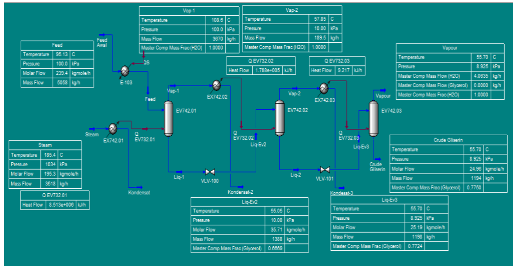
Gambar 1. Simulasi HYSYS pada Kondisi Proses secara prktis Kondisi operasi yang digunakan pada steam didapatkan berdasarkan data dari Steam Table untuk steam dengan tekanan 10,34 bar dan dilakukan perhitungan interpolasi
