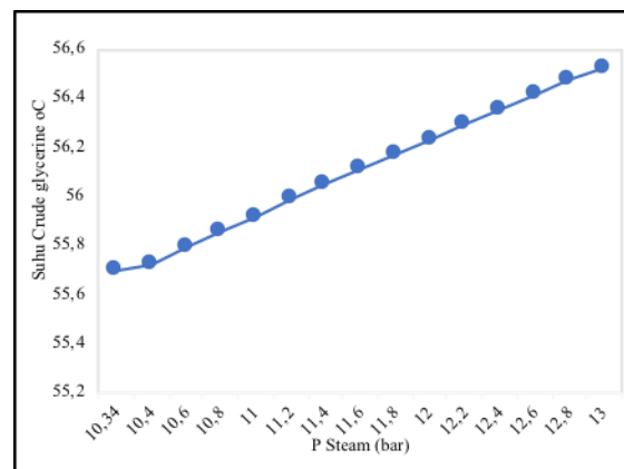
Grafik 6. Pengaruh Suhu Crude glycerine terhadap Penggunaan Berbagai Jenis Steam
