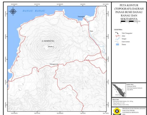
Gambar 4. Peta Kontur (Topografi) Daerah Panas Bumi Danau Ranau dan Sekitarnya
