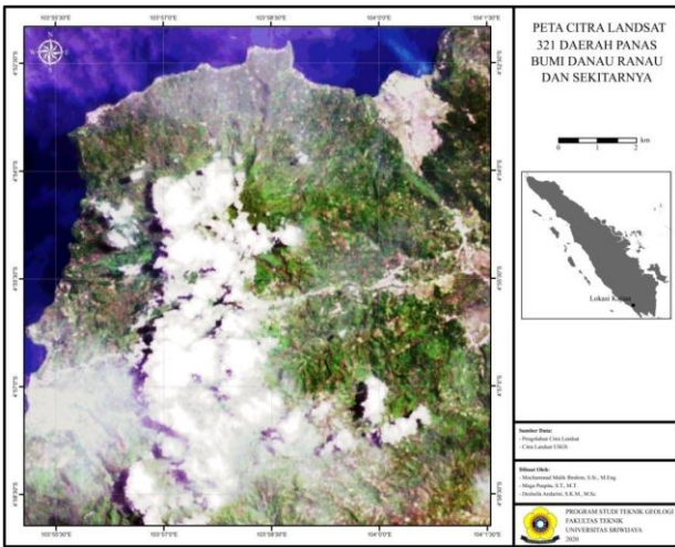
Gambar 1. Peta Citra Landsat 321 Daerah Panas Bumi Danau Ranau dan Sekitarnya
