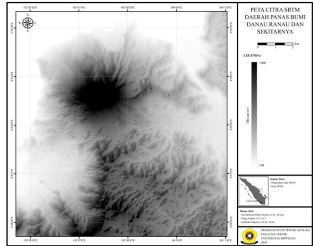
Gambar 3. Peta Citra SRTM Daerah Panas Bumi Danau Ranau dan Sekitarnya
