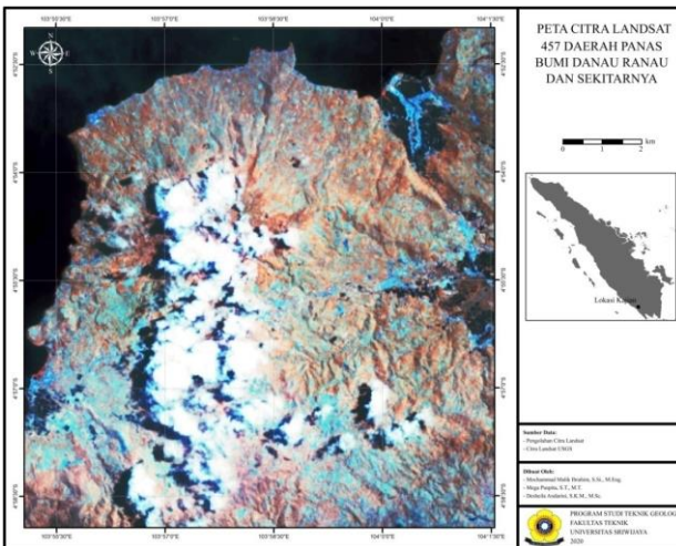
Gambar 2. Peta Citra Landsat 457 Daerah Panas Bumi Danau Ranau dan Sekitarnya
