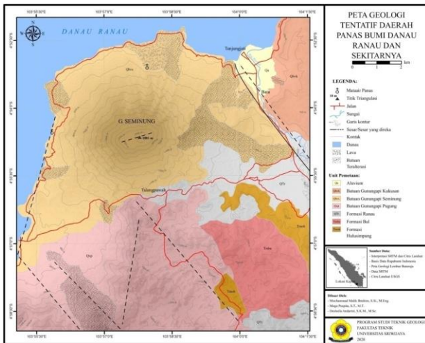
Gambar 5. Peta Geologi Daerah Panas Bumi Danau Ranau dan Sekitarnya
