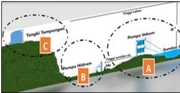
Gambar 5 Konsep Rancangan Pompa Vachydrum.
