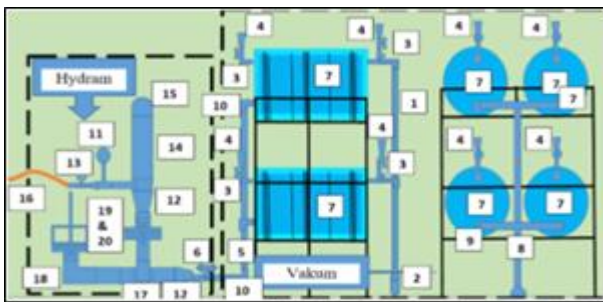
Gambar 6. Skema Rancangan Pompa Vachydrum.
