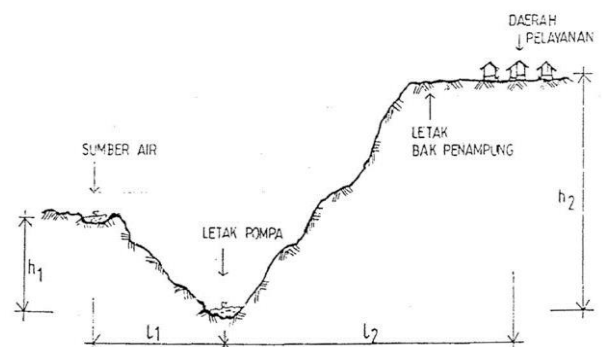
Gambar 4. Faktor-faktor pendukung kondisi lapangan dalam perencanaan pompa hidram.
