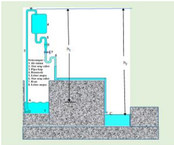
Gambar 3 Kondisi aliran yang dapat mengalir secara gravitasi.
