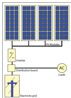
Gambar 2 Skema PLTS on-grid
