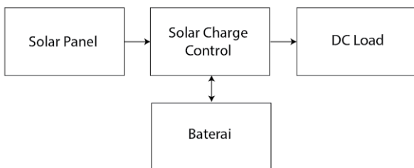
Gambar 6 Blok Diagram rangkaian PLTS
