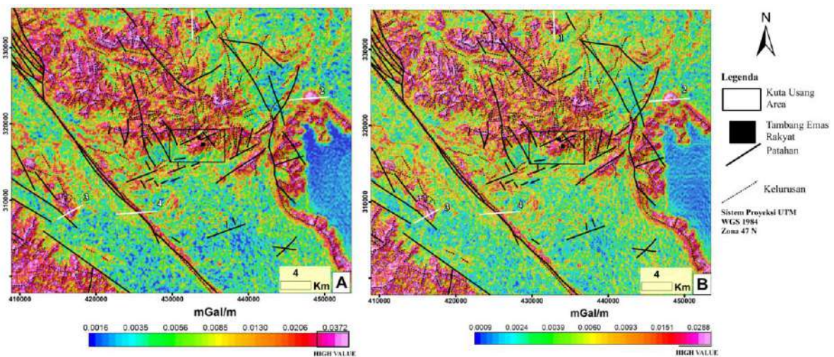
Gambar 3. Peta AS (A) dan Peta THD (B) dari Peta CBA. Keterangan: garis profil diterapkan pada intrusi granit (A), pusat vulkanik Kuartar (B), bukit gamping Paleozoik (C), dan Patahan Sumatera (D)
