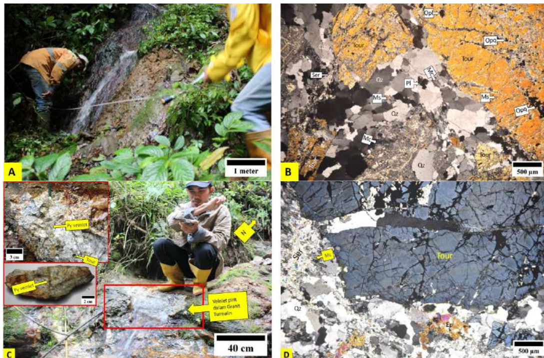
Gambar 8. Foto singkapan granit KU-04 (A dan B) dan KU-22 (C dan D) beserta fotomikrografnya. Singkatan: ser (serisit), mc (mikroklin), qz (kuarsa), py (pirit), opq (opak), ep (epidote), tour (turmalin).
