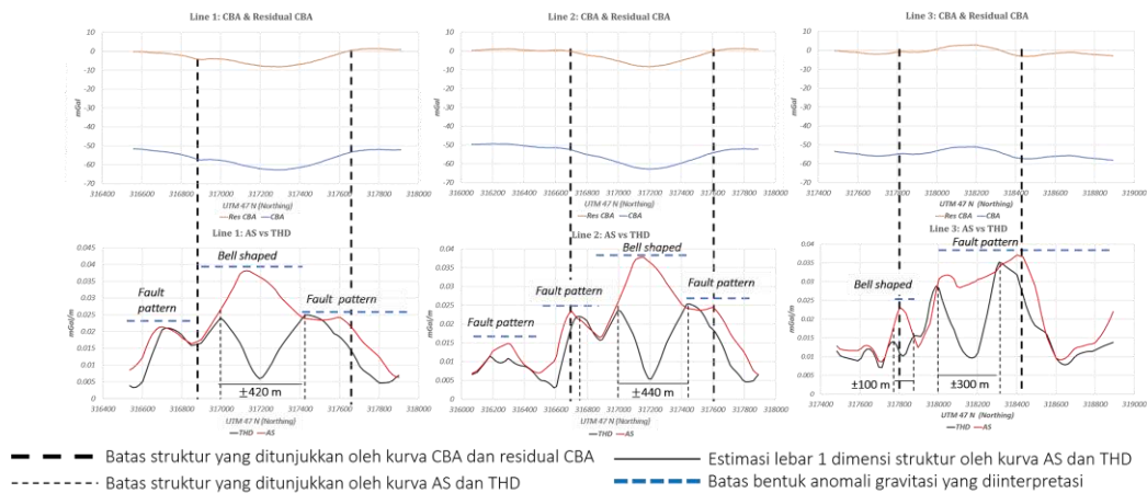
Gambar 7. Kurva CBA, residual CBA, AS, dan THD garis profil dari di area tambang rakyat Kuta Usang.
